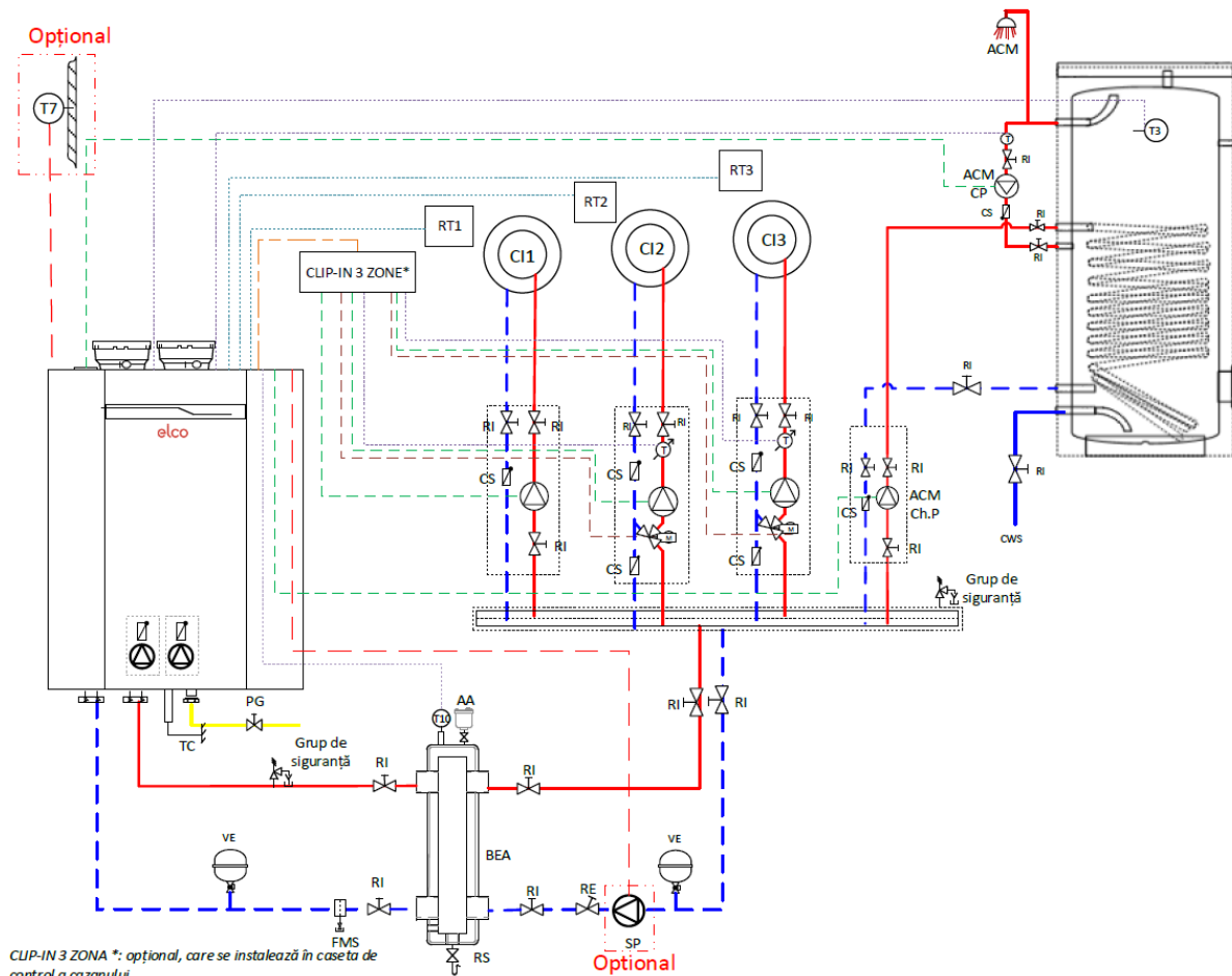
Schema hidraulică
